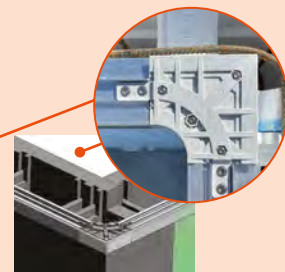
Uitgaande hoek
