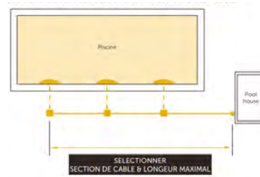
BEDRADINGSINSTRUCTIES SCHEMA - CONFIGURATIE 2
