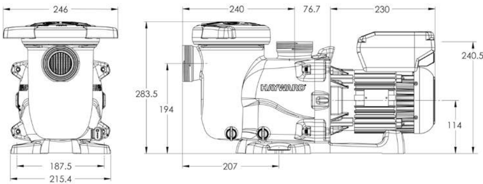
MAX-FLO™ XL VSTD
