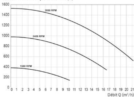
MAX-FLO™ XL VSTD
