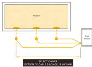
BEDRADINGSINSTRUCTIES SCHEMA - CONFIGURATIE 1
